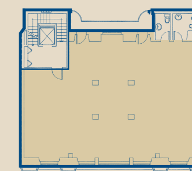
PISO 4 – 177 m 2
